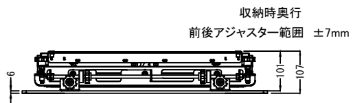
平面(収納時)
