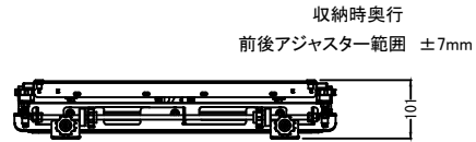
平面(収納時)
